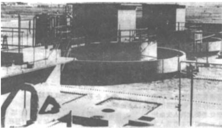
△ 我市第一座利用微生物日处理污水1400m 3 的污水处理装置，日前在垦利县炼油厂建成投产。经初步测试，达到国家规定的污水排放标准，日回收污油2吨以上。(曹玉松 曲志军 摄)
